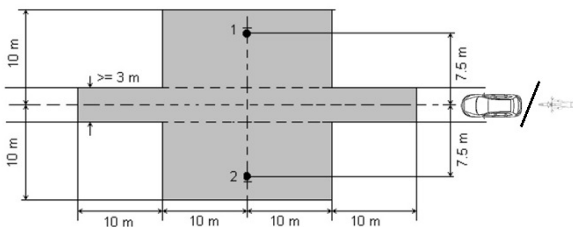
Figura 1 Diagrama de la pista de prueba
